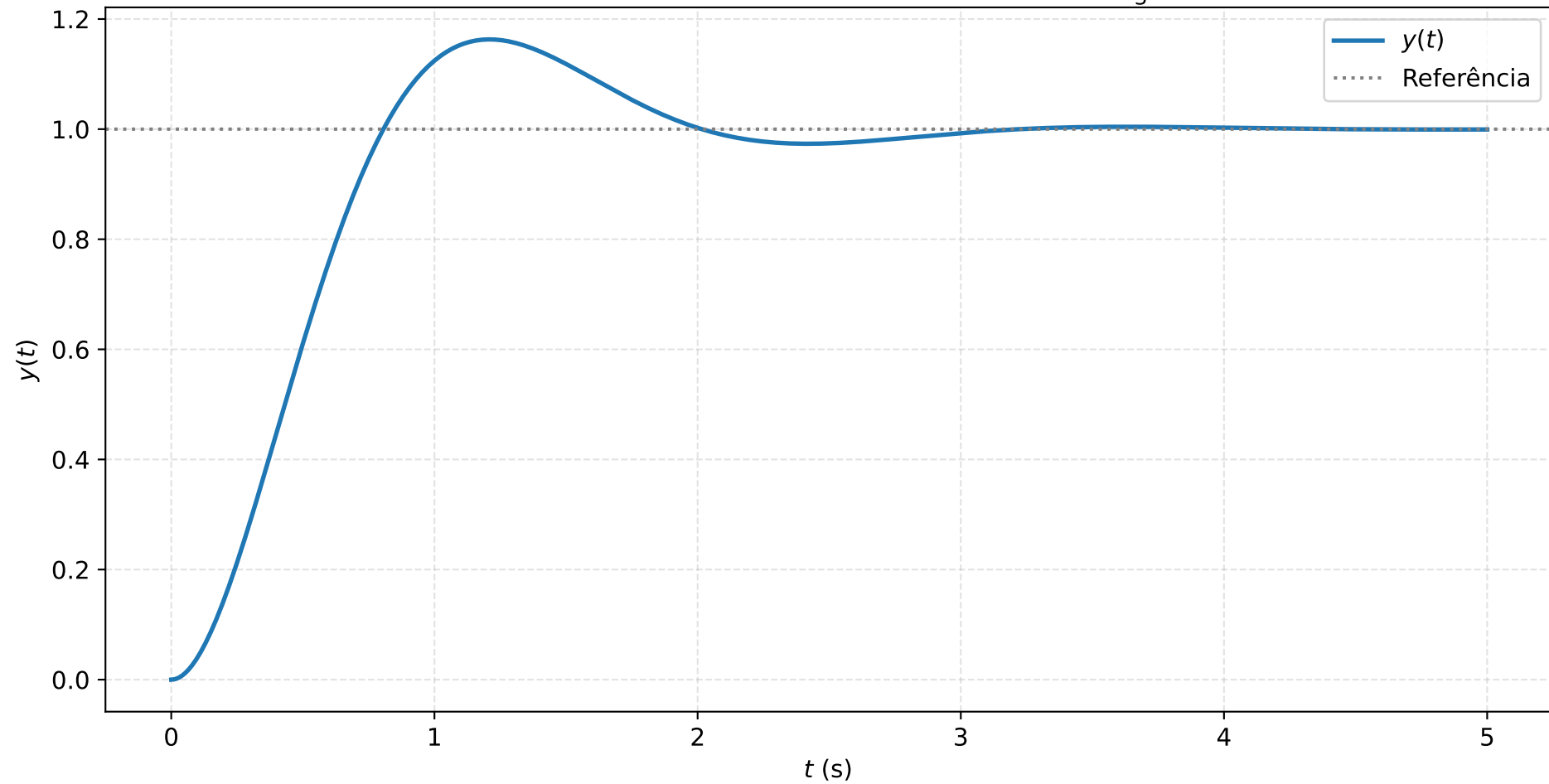
Questão B.6.15 --- Resposta ao degrau ( T_1 = 1 , T_2 = \frac{1}{3} , K = 0,3 )
